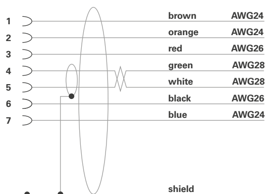
Pre-cabled receptacle 7 contacts (UR80)
